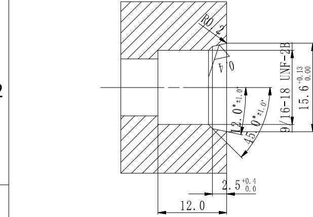
开孔尺寸
